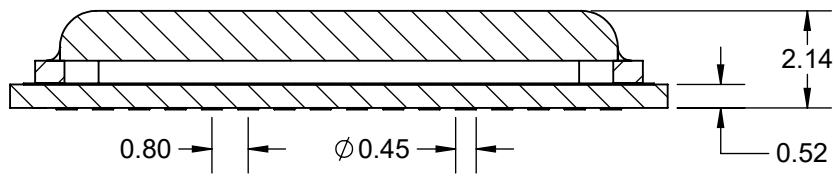
SECTION B-B SCALE 6 : 1
