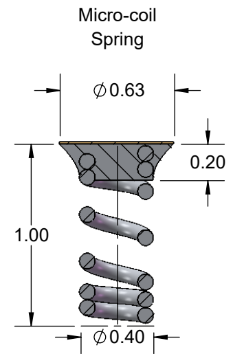
SECTION D-D SCALE 35 : 1
