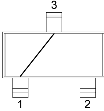
SOT723 - DC13 DWG 120313
