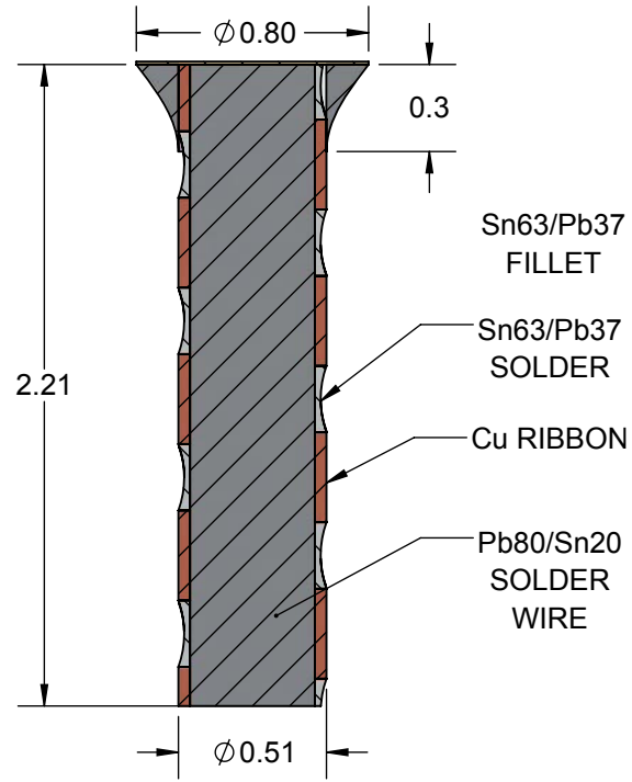
SECTION B-B SCALE 35 : 1
