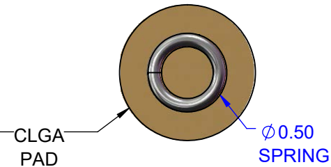
SECTION D-D SCALE 35 : 1
