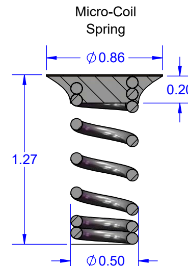
SECTION D-D SCALE 35 : 1
