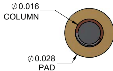
SECTION B-B SCALE 35 : 1
