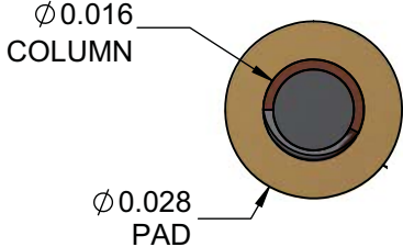
SECTION B-B SCALE 35 : 1
