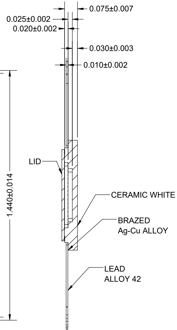
SECTION A-A SCALE 3 : 1
