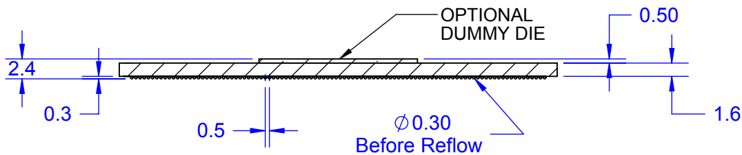
SECCION A-A
