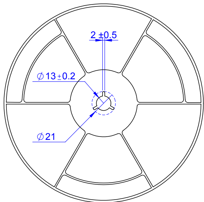
REEL DIMENSIONS
