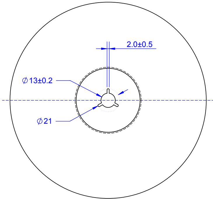
REEL DIMENSIONS
