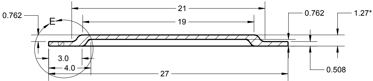
SECTION B-B SCALE 4 : 1
