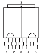
DC1245 D2PAK5
