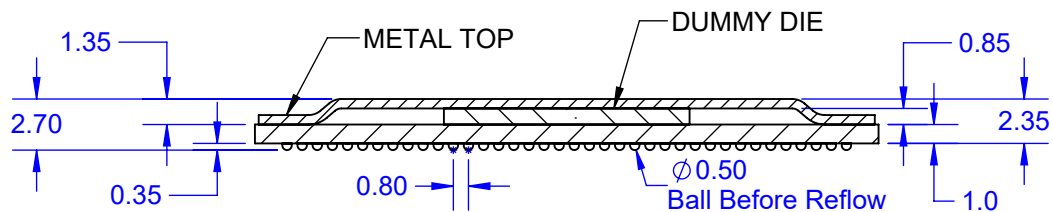
SECTION A-A
