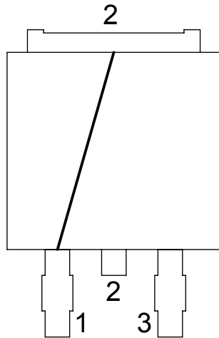
DPAK - DC12 D2PAK - DC12 DWG 120112
