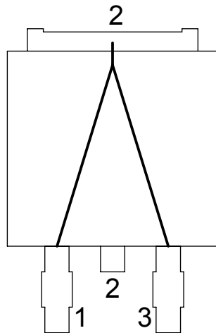
DPAK - DC123 D2PAK - DC123 DWG 121123
