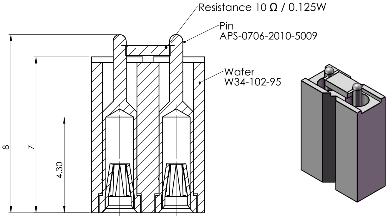
COUPE A-A
