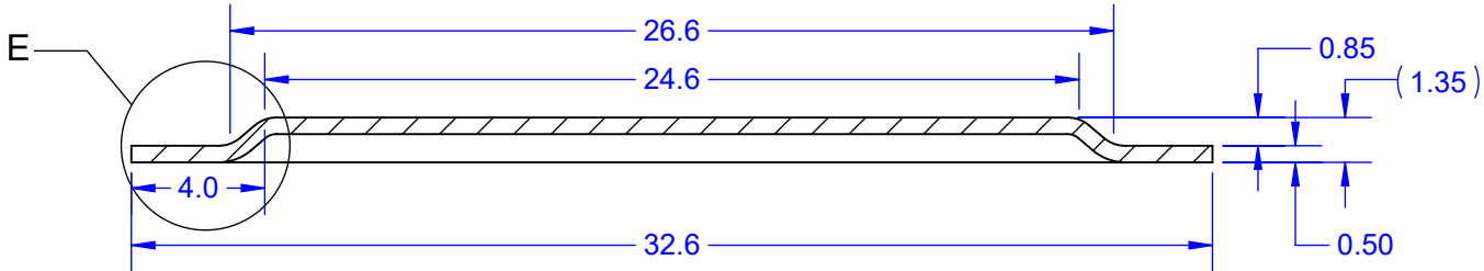
SECTION B-B SCALE 4 : 1
