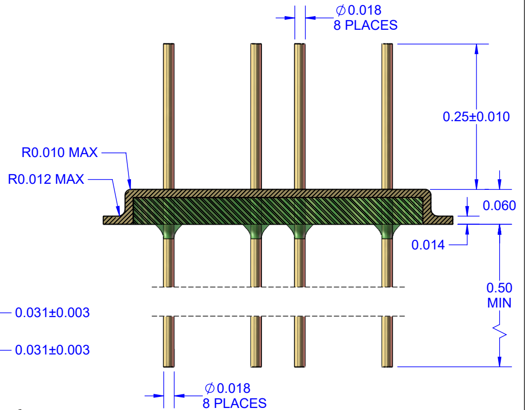
SECTION A-A SCALE 6 : 1
