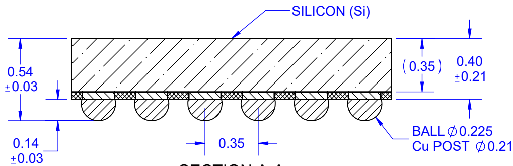
SECTION A-A SCALE 40 : 1
