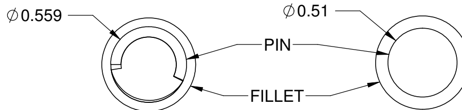
SECTION B-B SCALE 35 : 1
